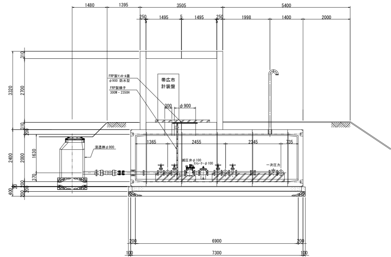
B-B断面図
