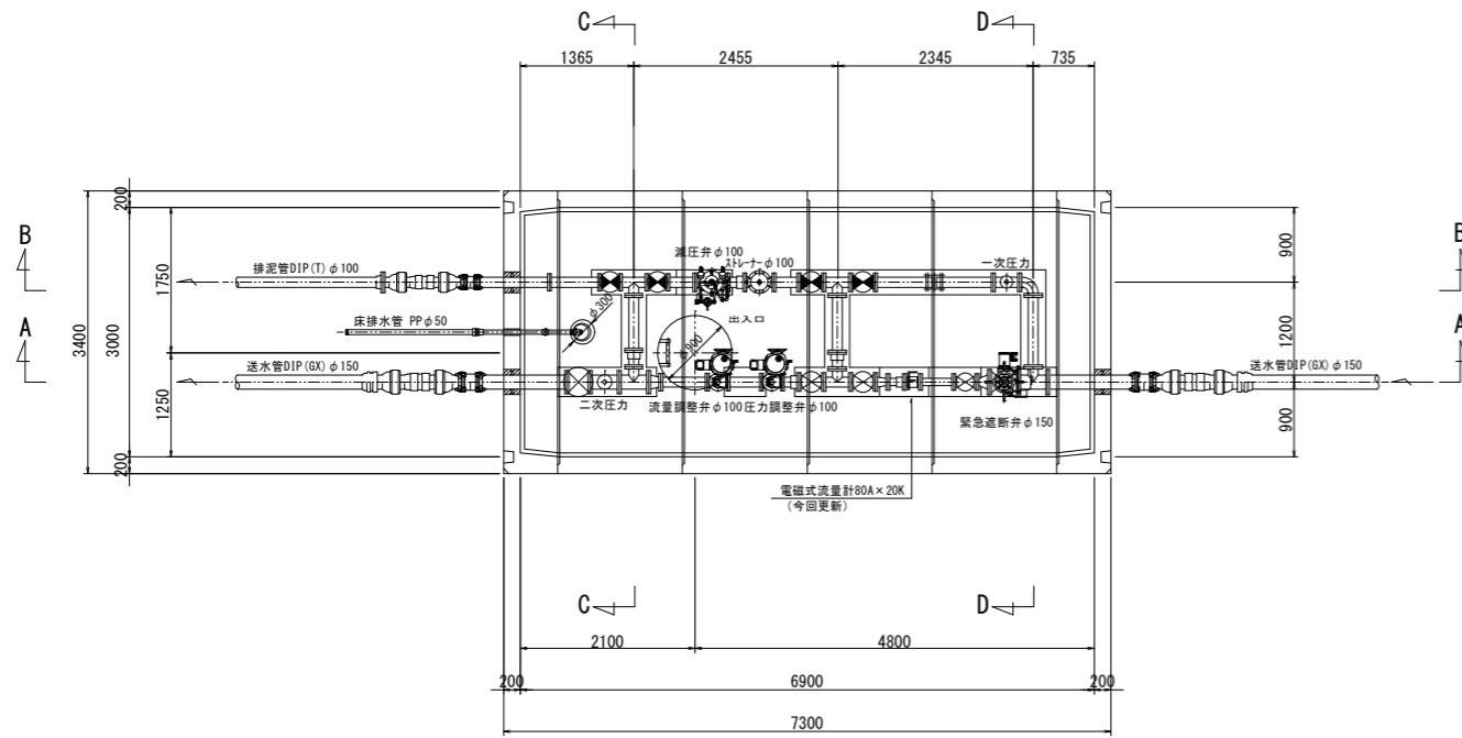
地下平面図
