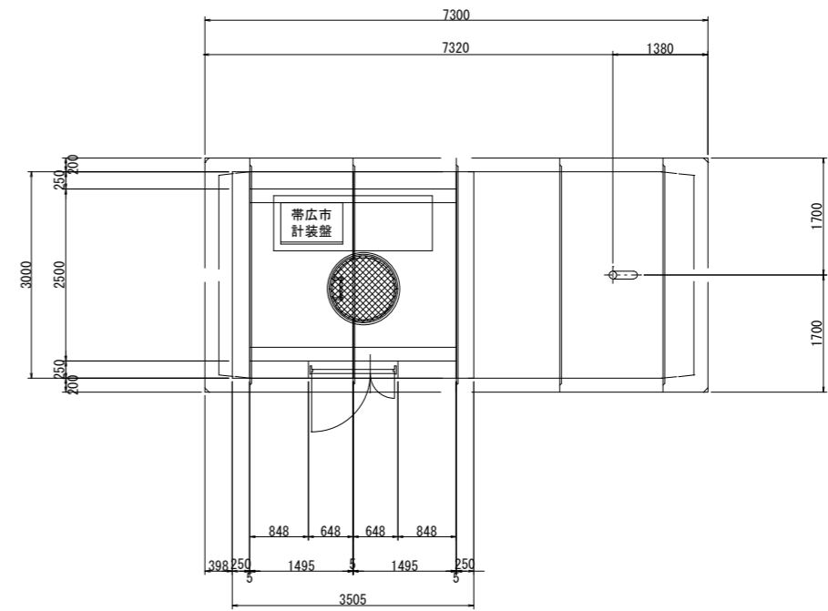
1F平面図
